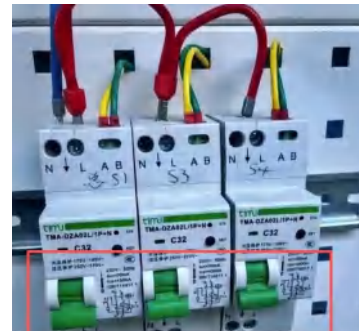
开合闸
