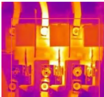
局部发热
