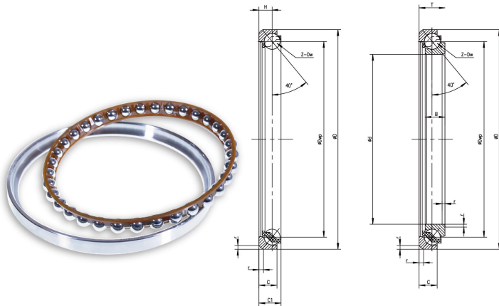
718B系列 RV減速器主軸承(角接觸球軸承)
